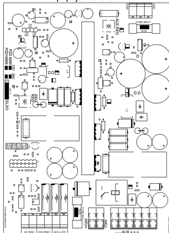
PZD6 připojení svorek
